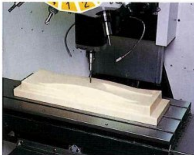
※加工プログラム提供:富士通株式会社殿 (Unigraphicsで作成) ワーク:パソコンフロントパネル 材質:ABS樹脂
