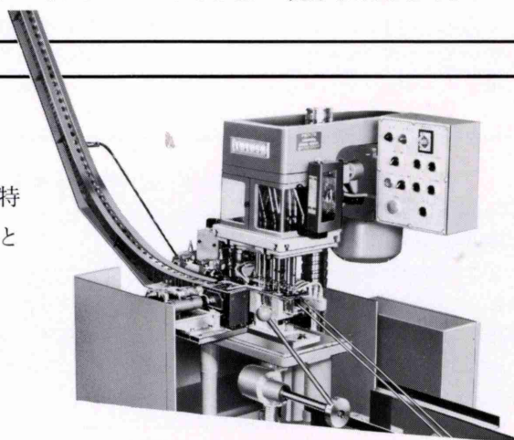
自動供給装置を取付けた全自動ネジ立て機
