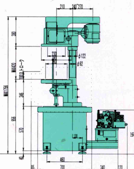
自動送り付外寸図
