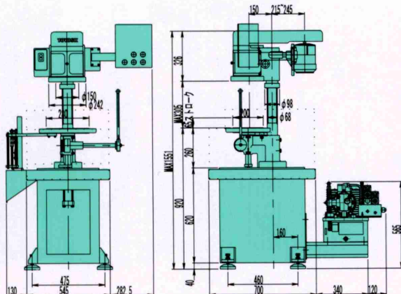
No.06 自動送り付外寸図
