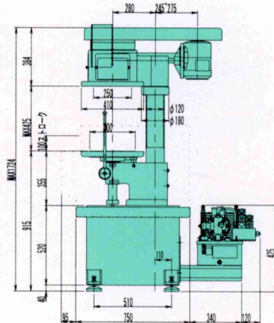
自動送り付外寸図
